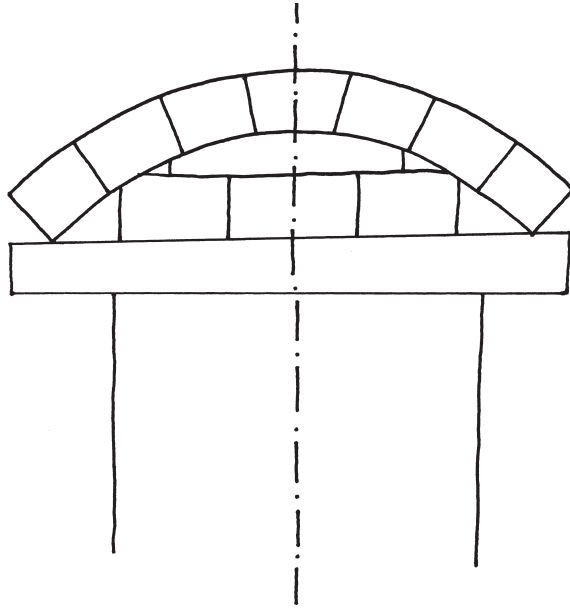
Arco de Descarga Discharging Arch
