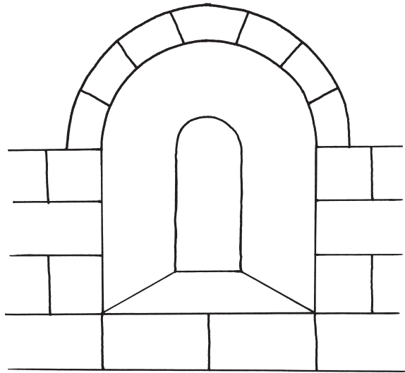
Arco Abocinado (Capialzado) Splayed Arch
