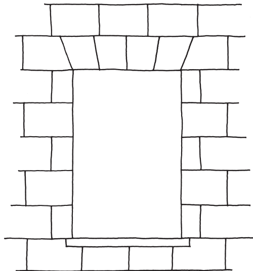
Arco Adintelado Flat Arch
